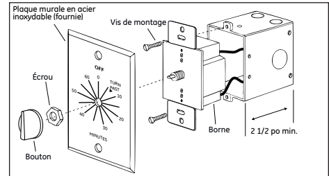
Montage de la plaque murale en acier inoxydable et du cadran Figure 4
