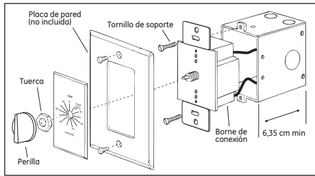
Instalación de la esfera y la placa de pared decorativa Figure 2
