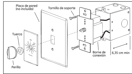
Instalación de la esfera y la placa de pared para interruptor de palanca Figure 3
